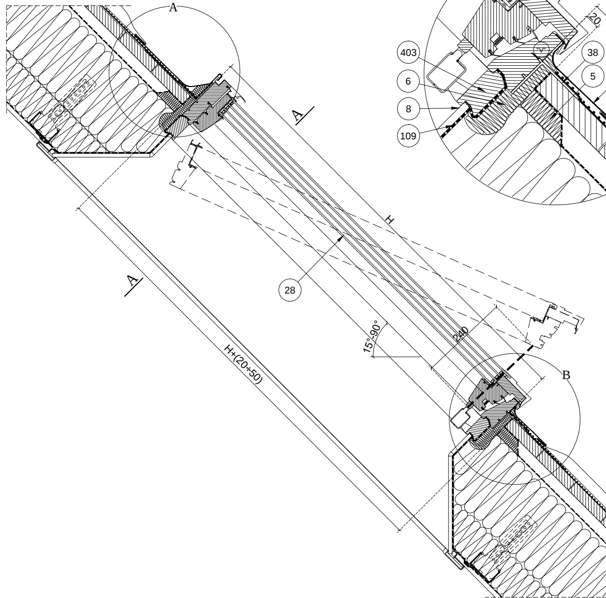
B - B
